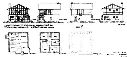
Figura 9 Vivienda familiar tipo F. Chalets sencillos.
