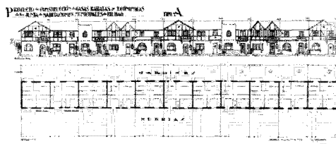
Figura 3 Vivienda familiar del tipo A constituida por chalets adosados.
