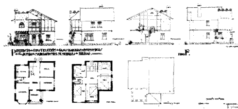
Figura 8 Vivienda familiar tipo F. Chalets sencillos.
