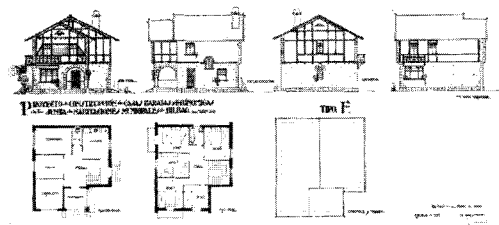
Figura 7 Vivienda familiar tipo F. Chalets sencillos. Obsérvense las diferencias con las dos siguientes.
