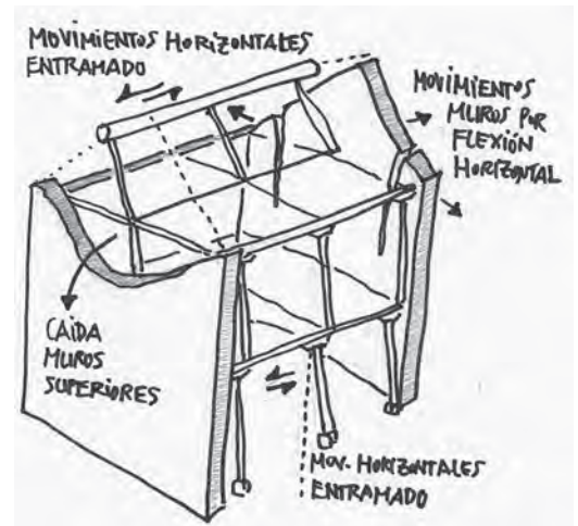
Figura 14 Dibujo de los daños habituales tras un sismo, sin llegar al colapso (Autores)
